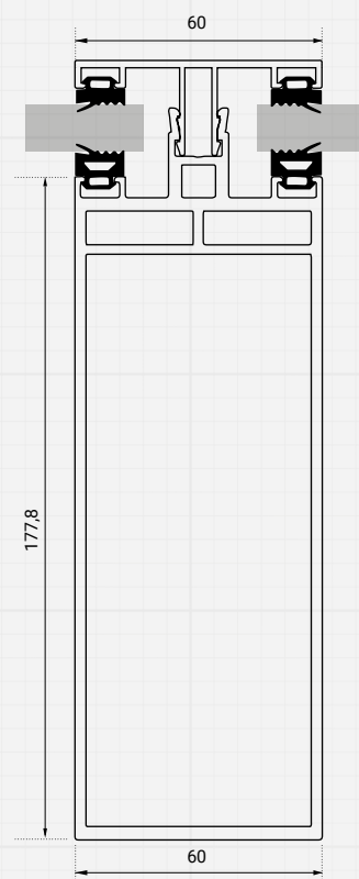
Querträger TR20
