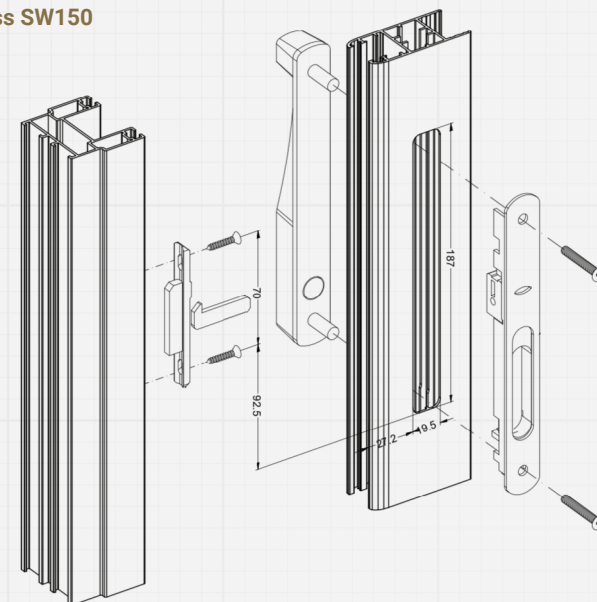
Seitenschloss SW150
