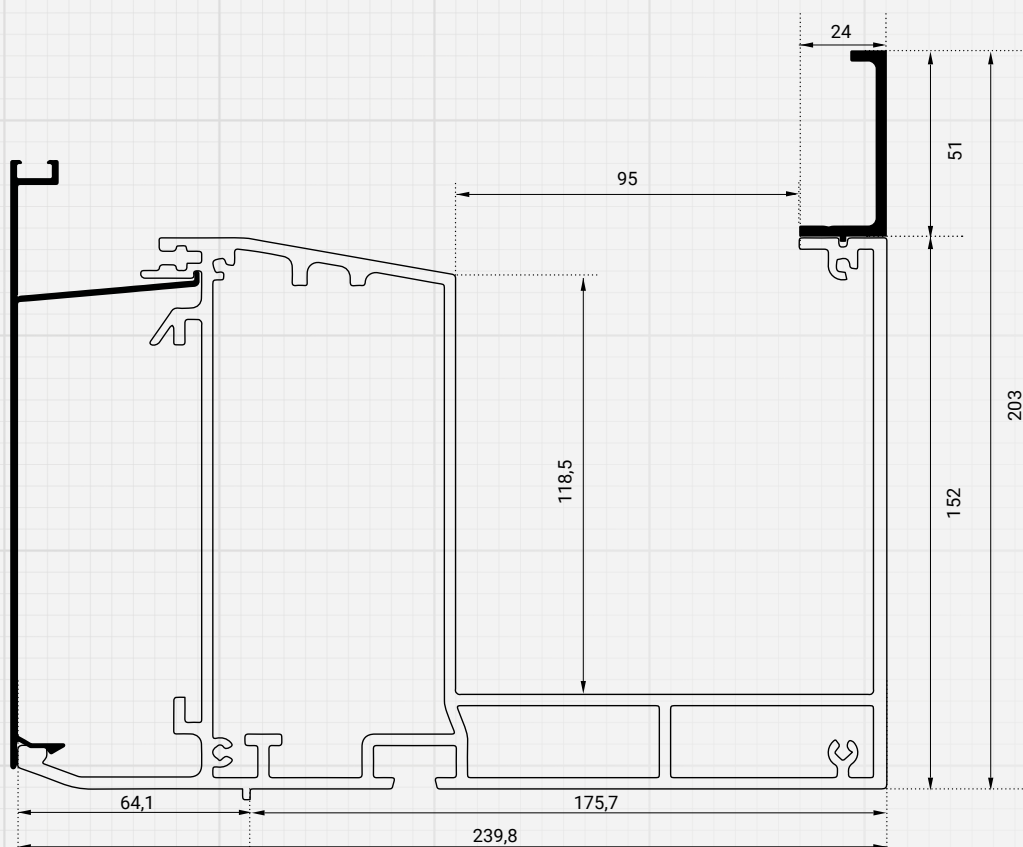
Rinne TR20 mit Aufsatzprofil und Klickblende
