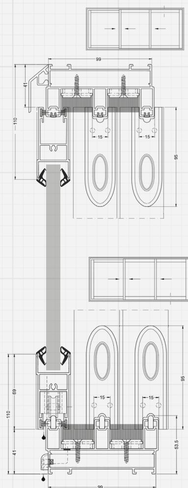
Ober- und Bodenschiene SW150 (3-spurig)
