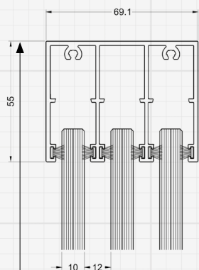
Ober- und Bodenschiene SW450 (3-Spurig)
