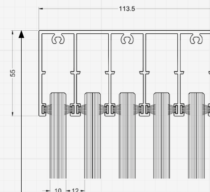
Ober- und Bodenschiene SW450 (5-Spurig)
