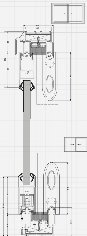
Ober- und Bodenschiene SW150 (2-spurig)
