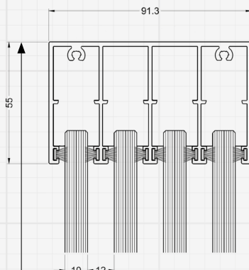
Ober- und Bodenschiene SW450 (4-Spurig)
